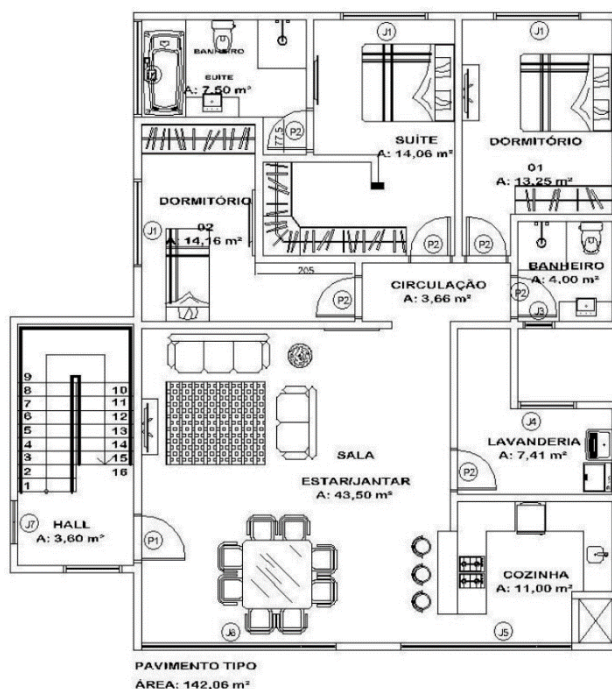
Figura 2 - Planta baixa pavimento tipo
