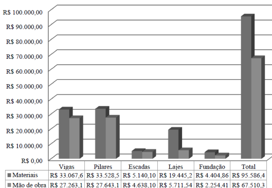
Gráfico 2 – Etapas construtivas de aço
