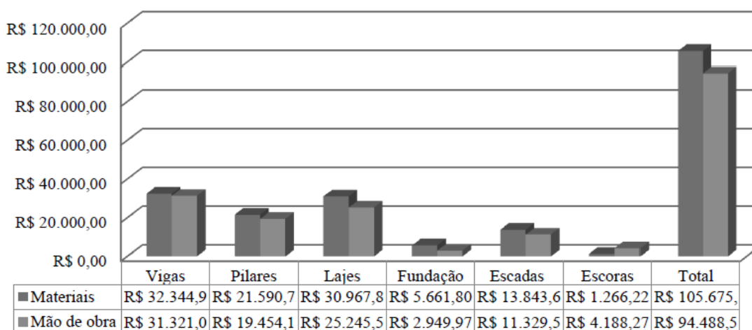
Gráfico 1 – Etapas construtivas de concreto armado
